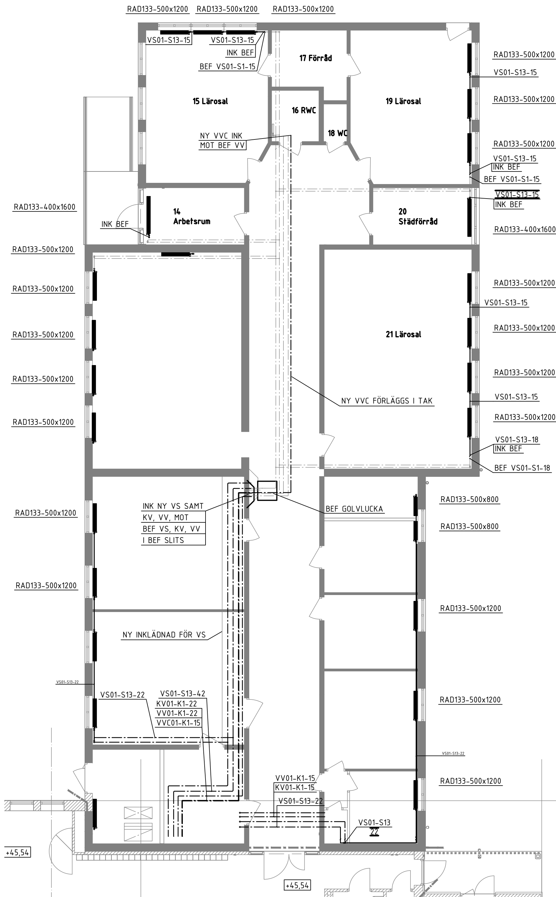
RÖRINSTALLATIONER SKALA 1:100
