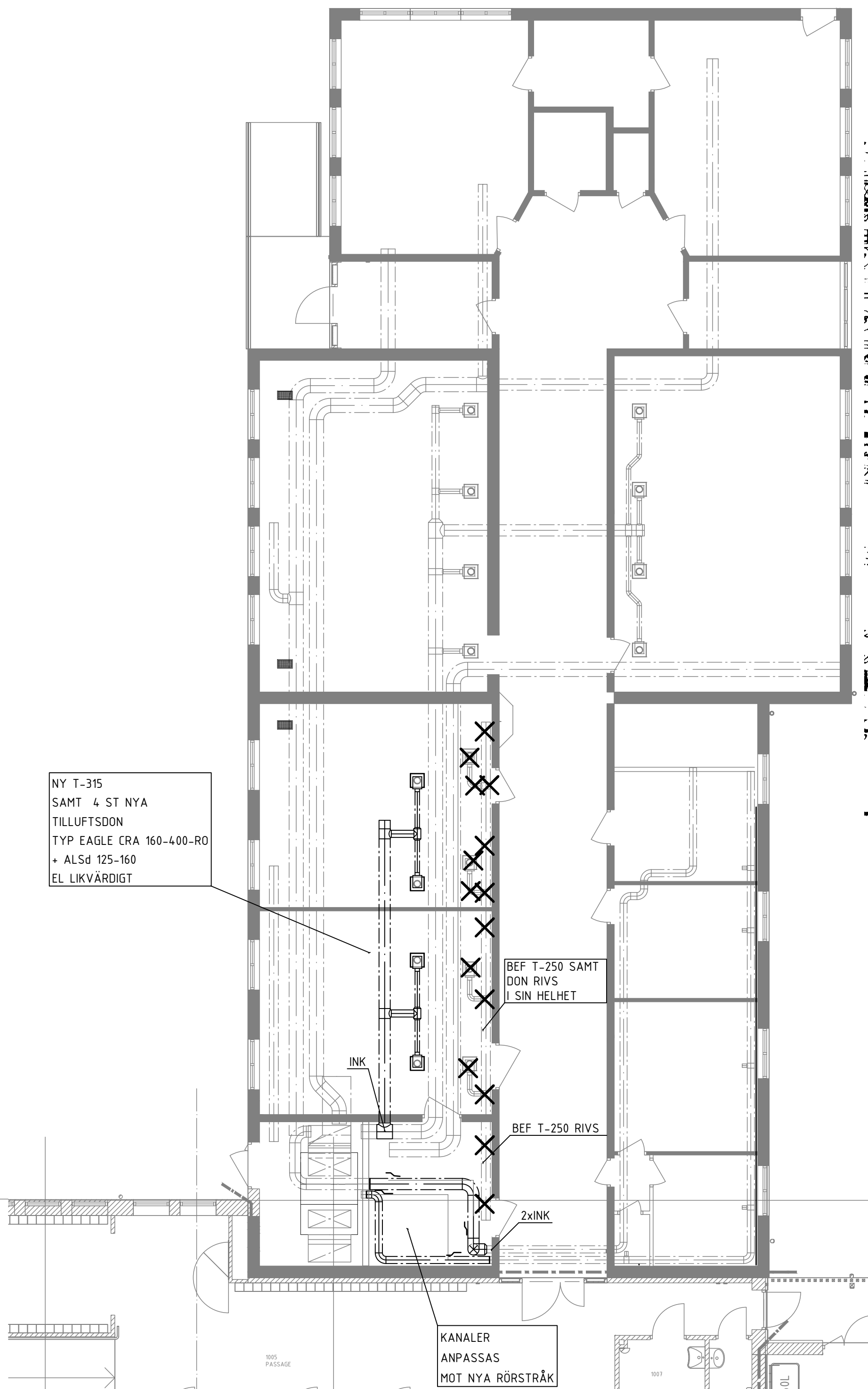
LUFTBEHANDLINGSINSTALLATIONER SKALA 1:100
